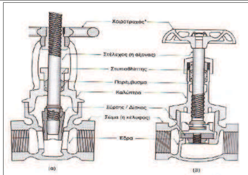
Τομή συρταρωτής (α) και σφαιρικής (β) βαλβίδας.
