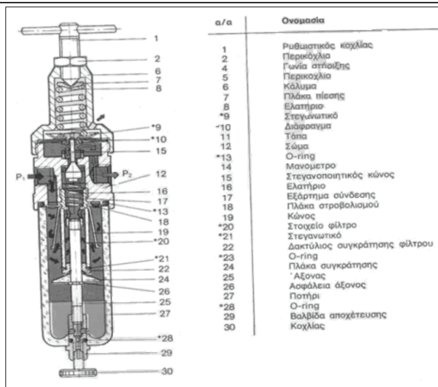
Φίλτρο και βαλβίδα ρύθμισης πίεσης
