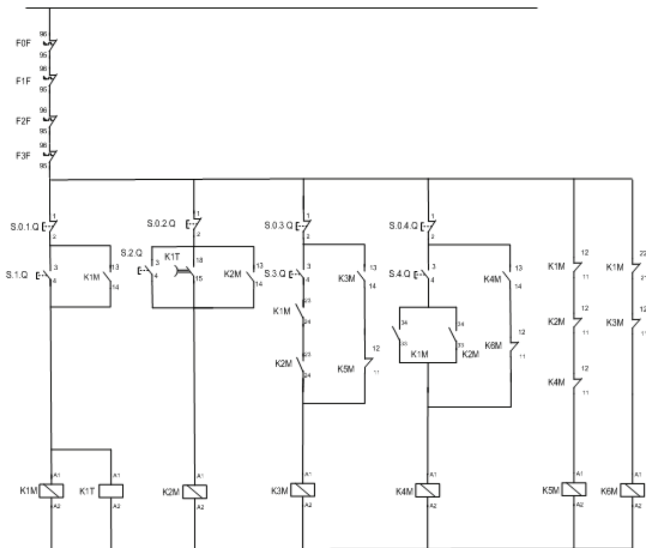
Σχήμα 2. Κύκλωμα αυτοματισμού
