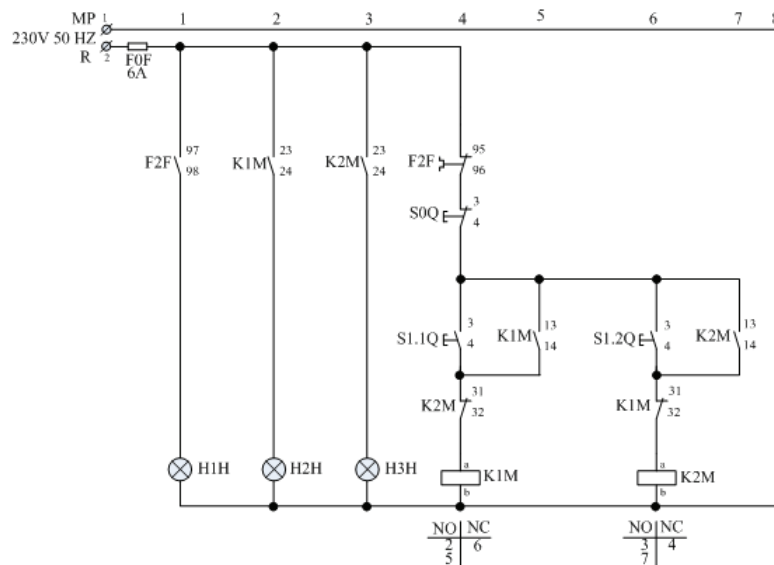
Σχήμα 2. Κύκλωμα Αυτοματισμού
