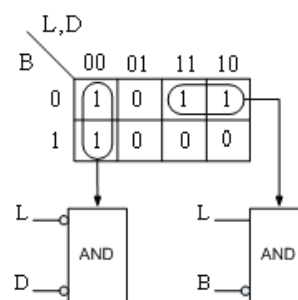
Σχήμα 6. Πίνακας αληθείας
