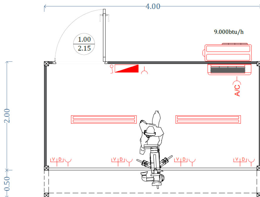
Εικόνα 3: Κάτοψη οικίσκου
